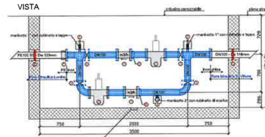
DETTAGLIO CAMERA 1:20
